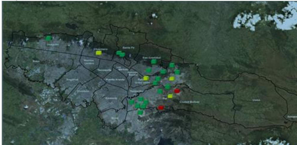
Mapa 37. Ubicación de las obras de mitigación construidas entre 2016-2019
