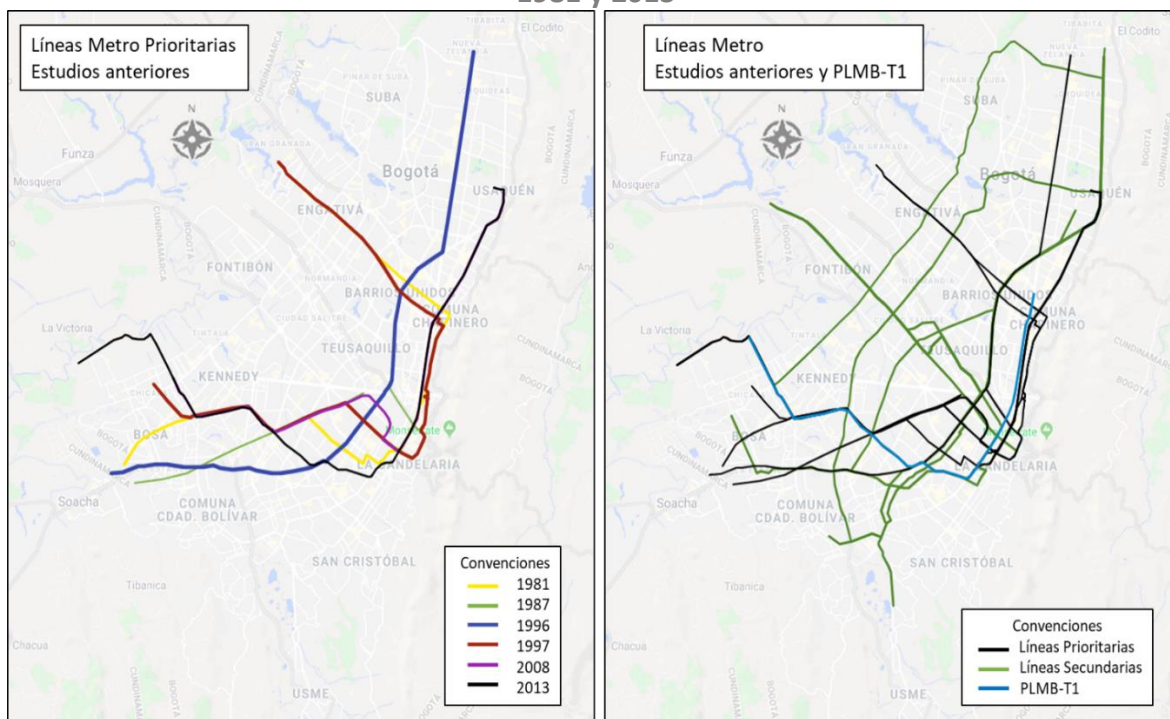
Mapa 64. Consolidado de trazados de líneas de metro según estudios realizados entre 1981 y 2013
