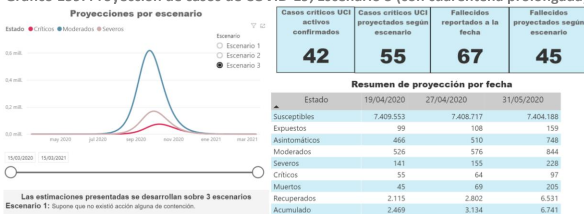
Gráfico 159. Proyección de casos de COVID-19, Escenario 3 (con cuarentena prolongada)
