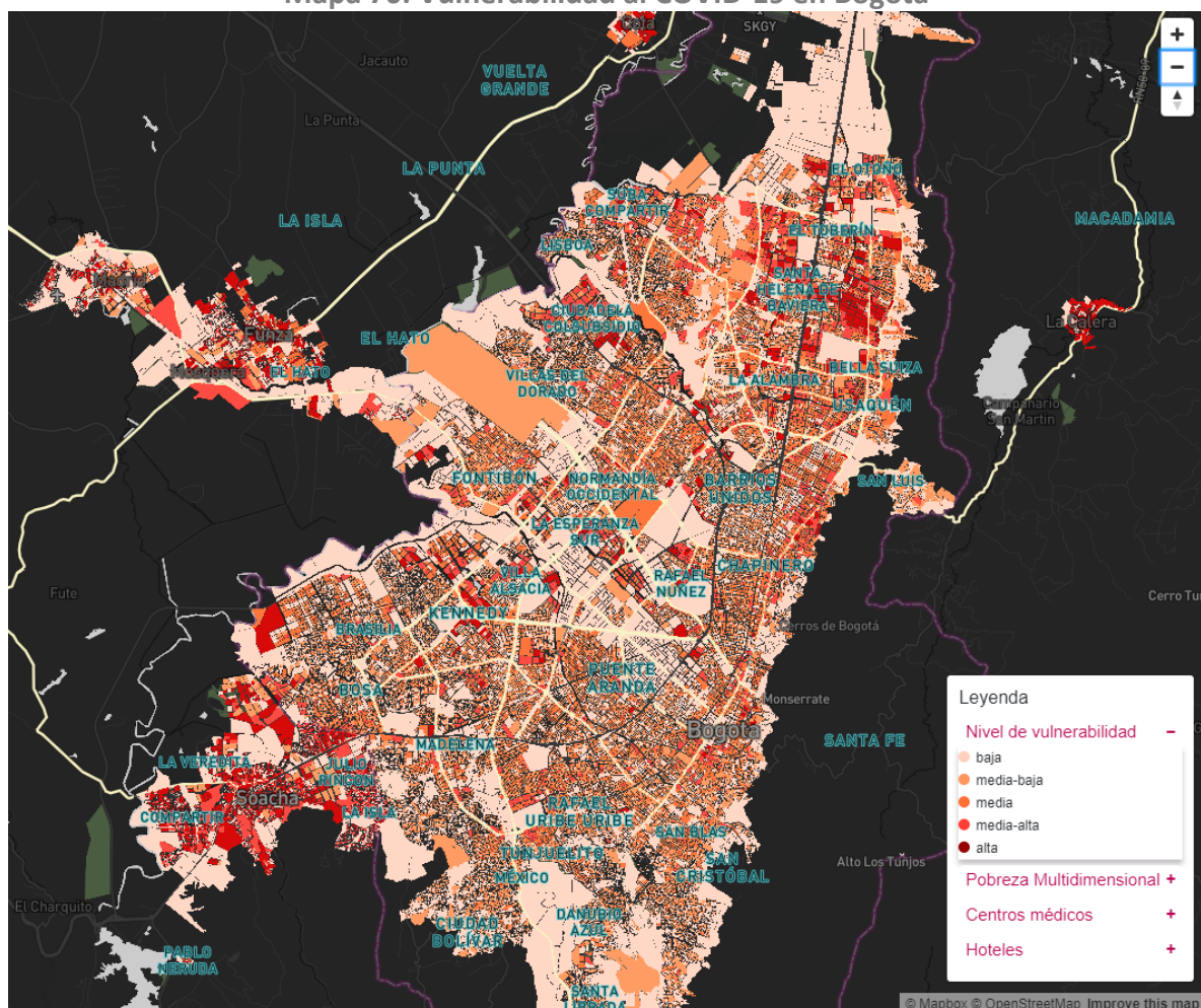
Mapa 70. Vulnerabilidad al COVID-19 en Bogotá
