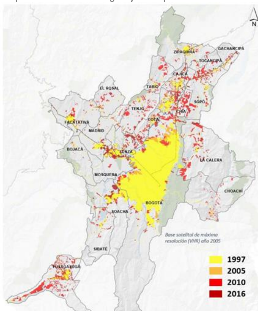
Mapa 32. Huella urbana Bogotá y municipios aledaños 1997-2016
