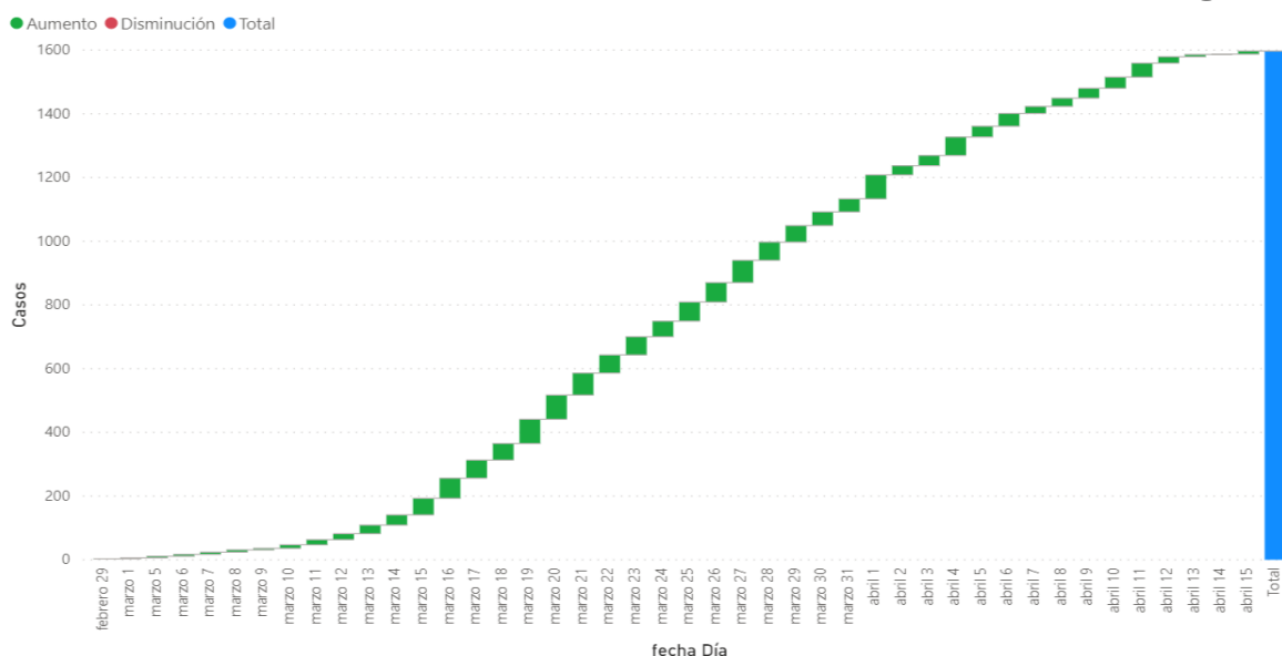
Gráfico 156. Curva acumulada de casos diarios confirmados de COVID-19 en Bogotá
