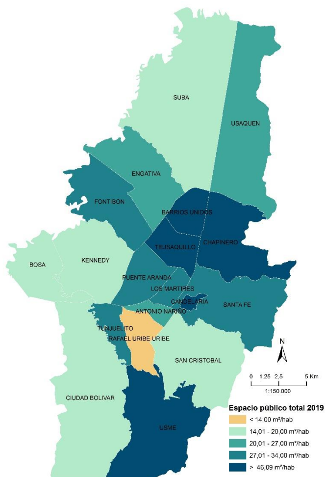
Mapa 59. Espacio público total, 2019
