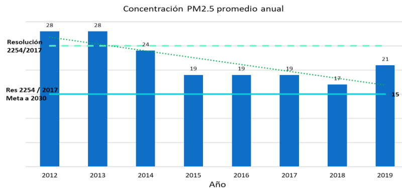
Gráfico 96. Concentración PM2.5 promedio anual
