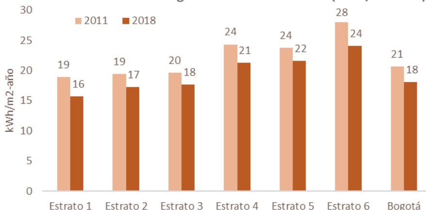
Gráfico 83. Consumo energía eléctrica residencial (kWh/m 2 -año)
