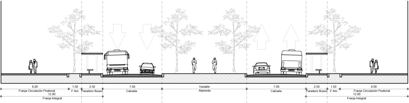
SECCIÓN PARADERO DE BUSES
