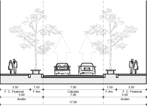
SECCION TIPO
