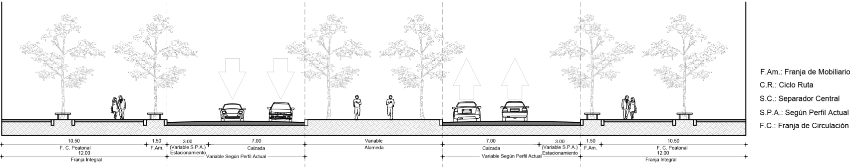
SECCIÓN ESTACIONAMIENTO EN VÍA
