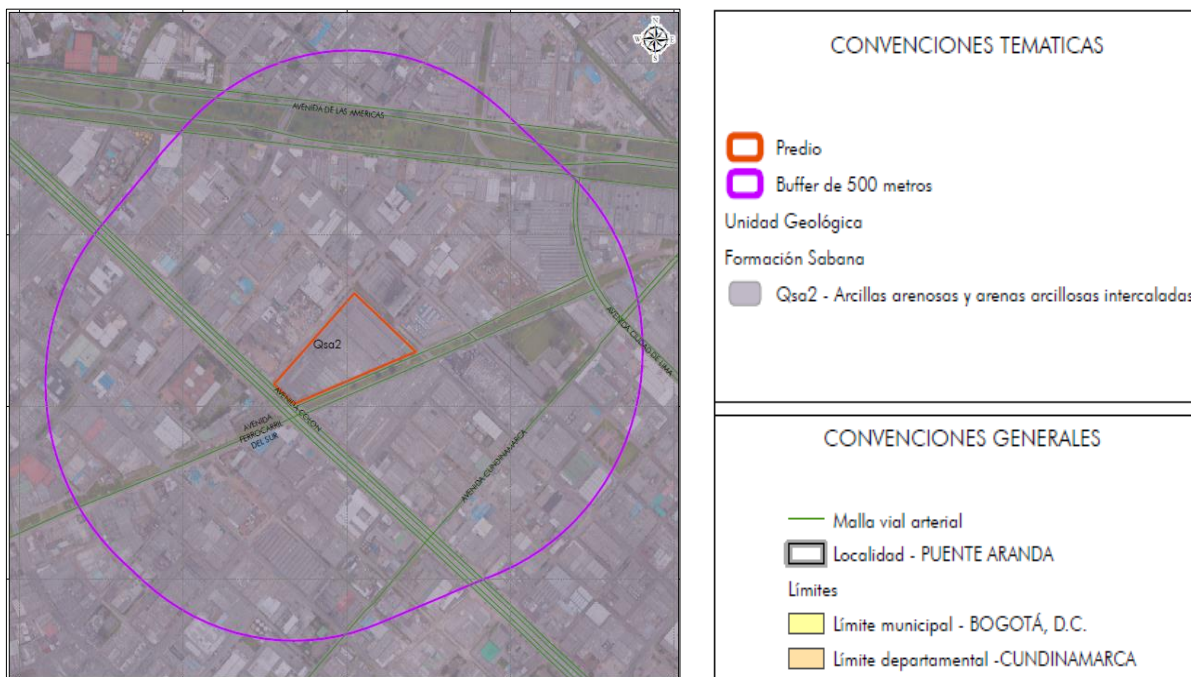
Figura 5-4. Geología del predio en un buffer de 500 m
