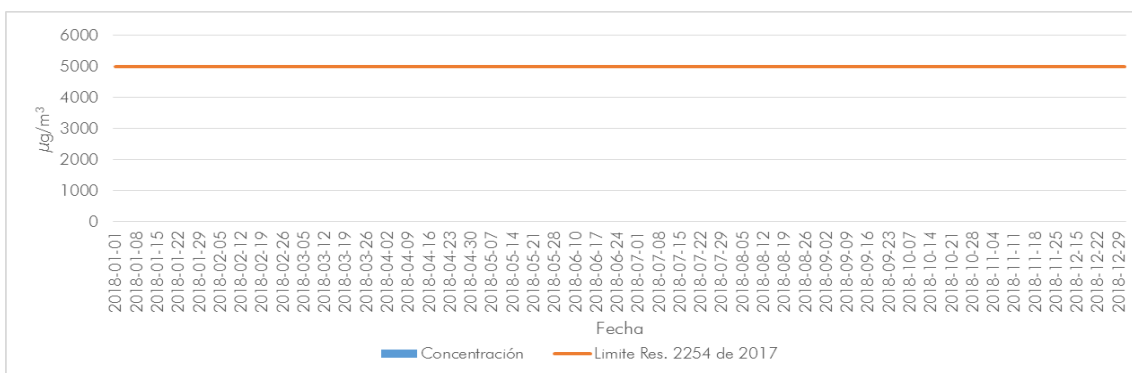
Gráfico 4-8. Concentraciones de Monóxido de Carbono CO estación Puente Aranda año 2018 – 8 horas
