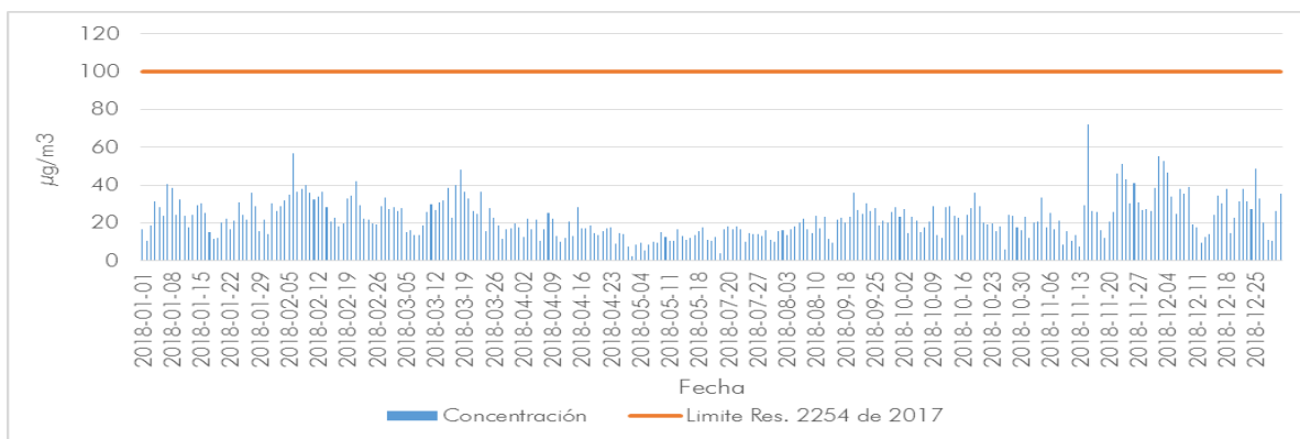
Gráfico 4-5. Concentraciones de ozono O_3 estación Puente Aranda año 2018 – 8 horas
