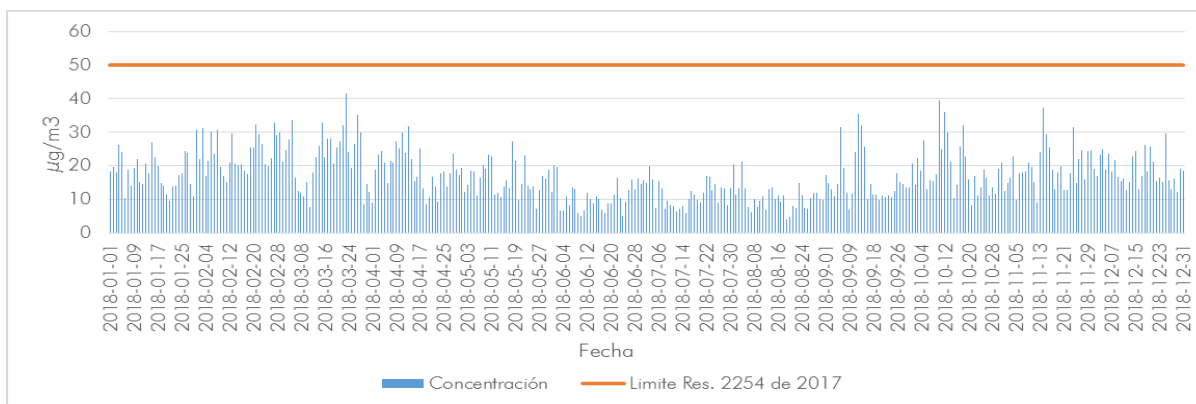
Gráfico 4-4. Concentraciones de PM 2.5 estación Puente Aranda año 2018 – 24 horas
