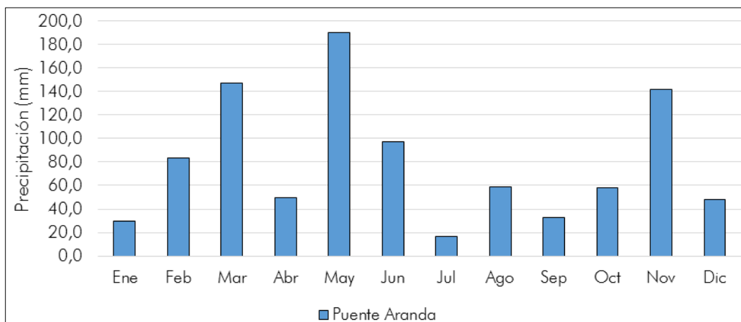
Gráfico 4-2 Precipitación mensual estación Puente Aranda – año 2017
