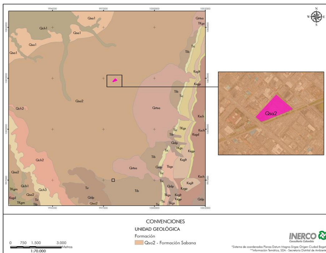
Figura 4-1 Geología local del área de intervención
