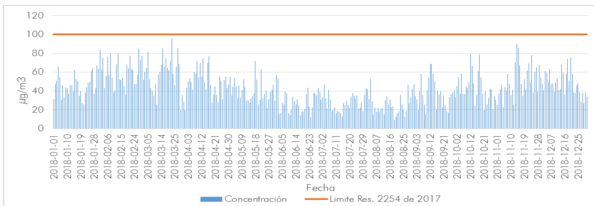
Gráfico 4-3. Concentraciones de PM 10 estación Puente Aranda año 2018 – 24 horas
