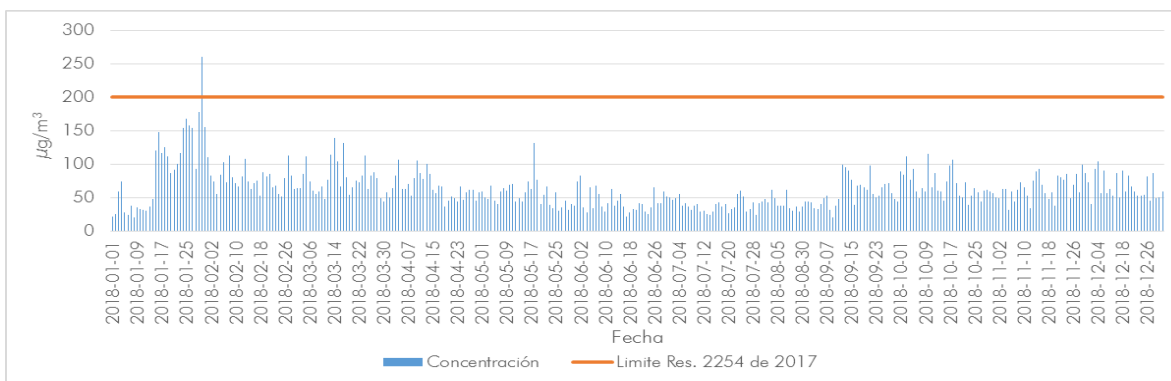
Gráfico 4-7. Concentraciones de Dióxido de Nitrógeno NO 2 estación Puente Aranda año 2018 – 1 hora
