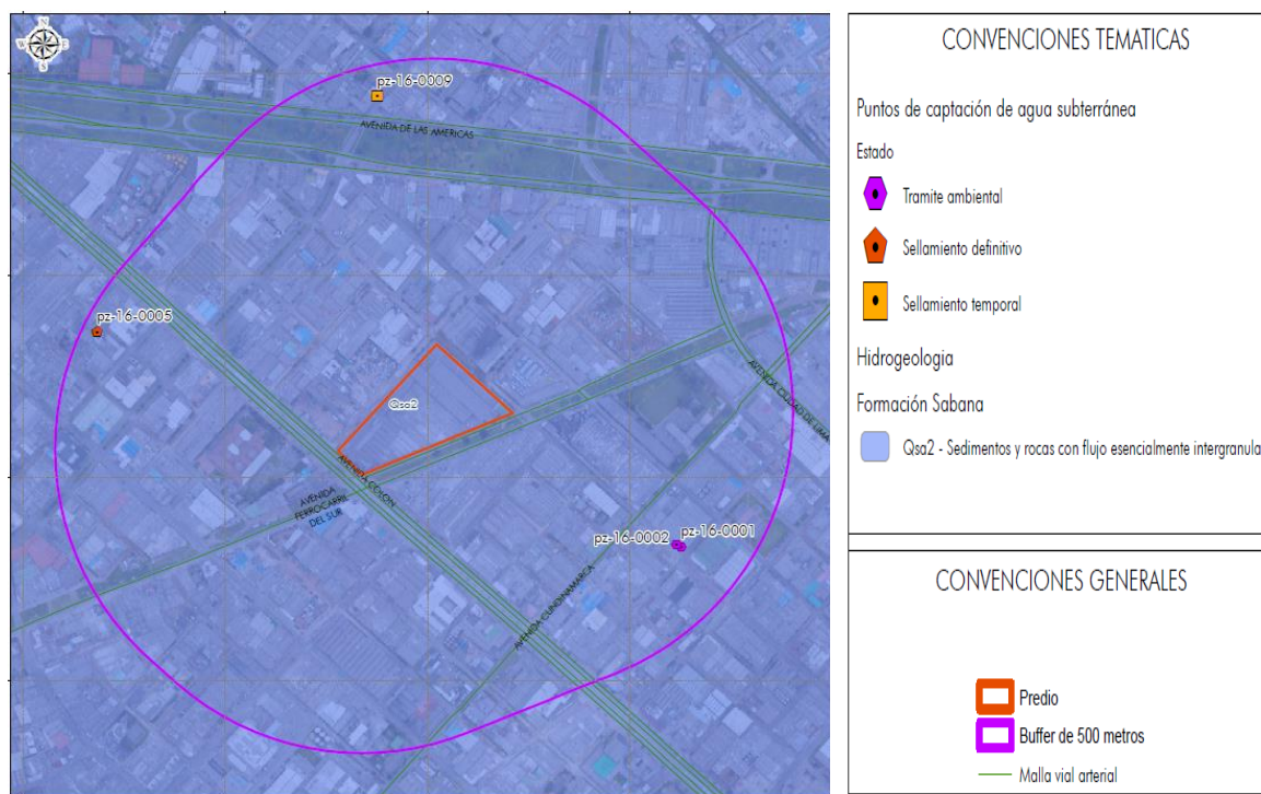
Figura 5-5 Hidrogeología del predio en un buffer de 500 m
