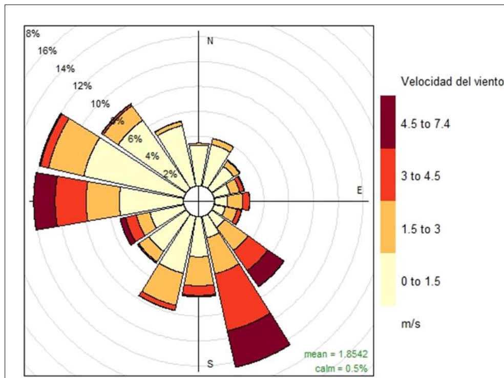
Figura 4-5 Rosa de los vientos estación Puente Aranda
