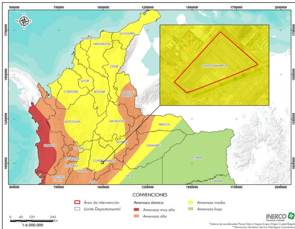
Figura 4-2 Amenaza sísmica en el área de intervención
