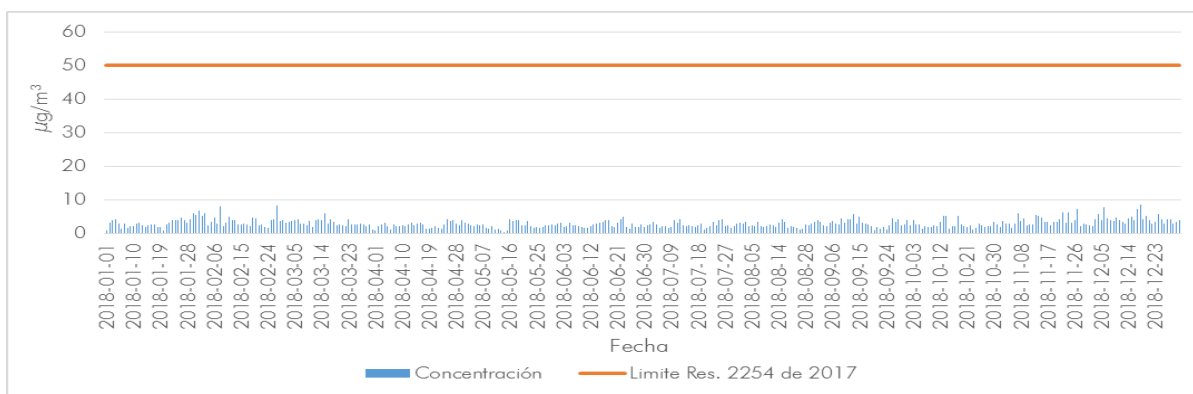
Gráfico 4-6. Concentraciones de Dióxido de Azufre SO_2 estación Puente Aranda año 2018 – 24 horas
