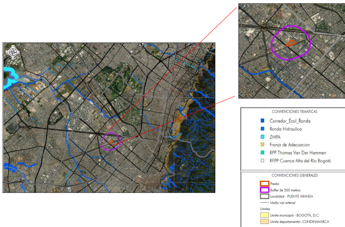
Figura 5-3 Hidrología del predio en un buffer de 500 m
