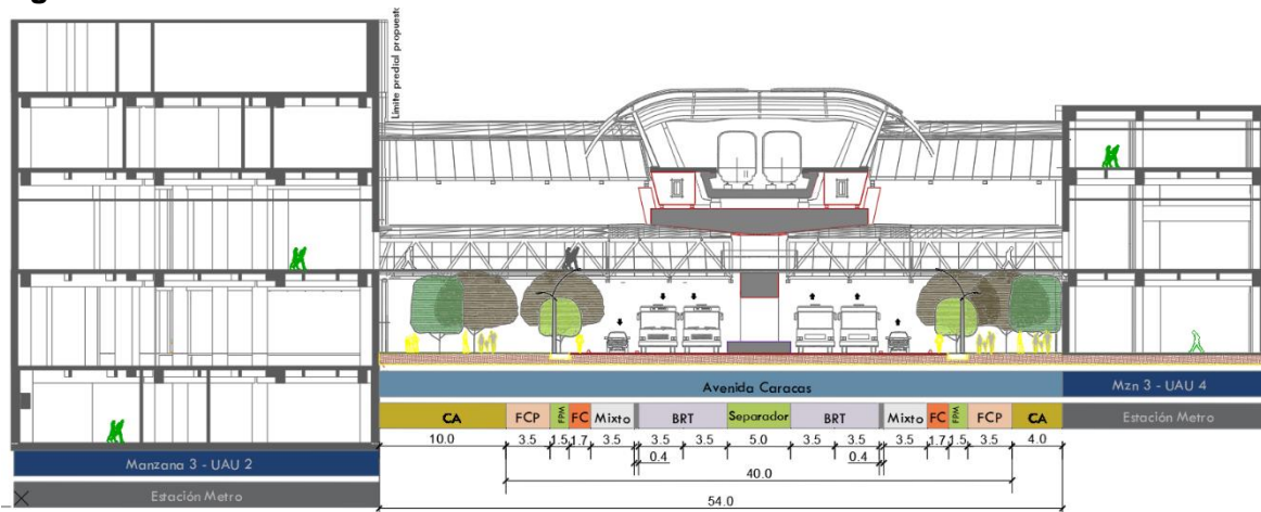
Figura 6-30. Sección transversal PLMB en el área de influencia
