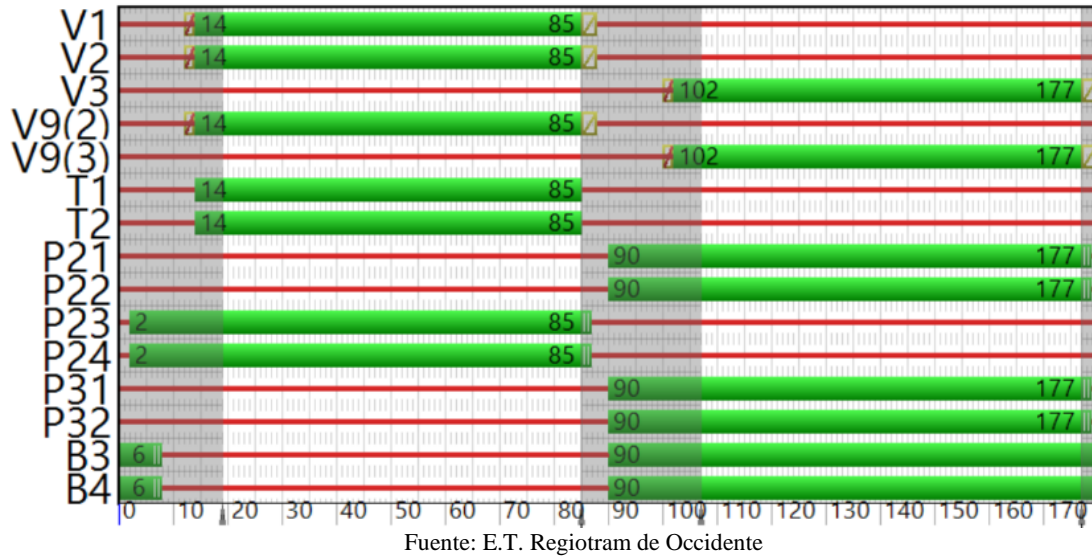
Figura 6-28. Planeamiento semafórico, Carrera 17 x Calle 24 de acuerdo al E.T. Regiotram de Occidente
