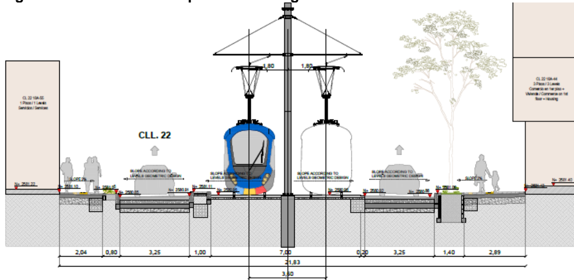
Figura 6-27. Perfil Calle 22 por trazado Regiotram
