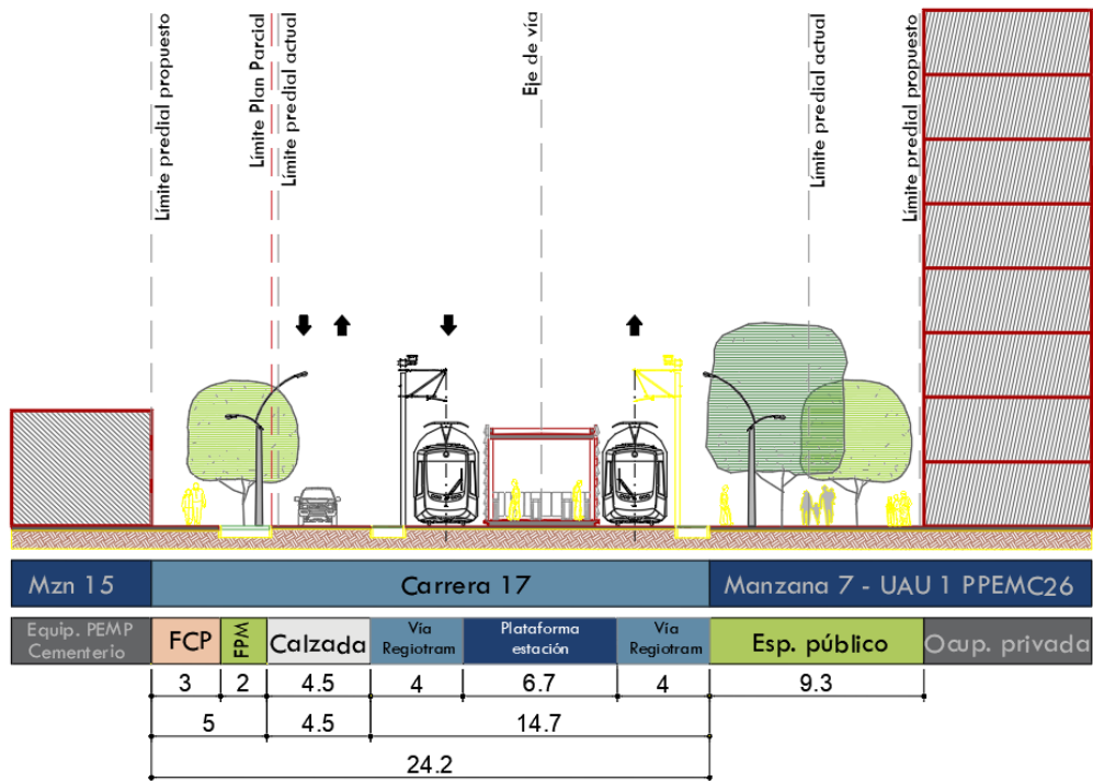
Figura 6-26. Perfil Carrera 17 por trazado Regiotram
