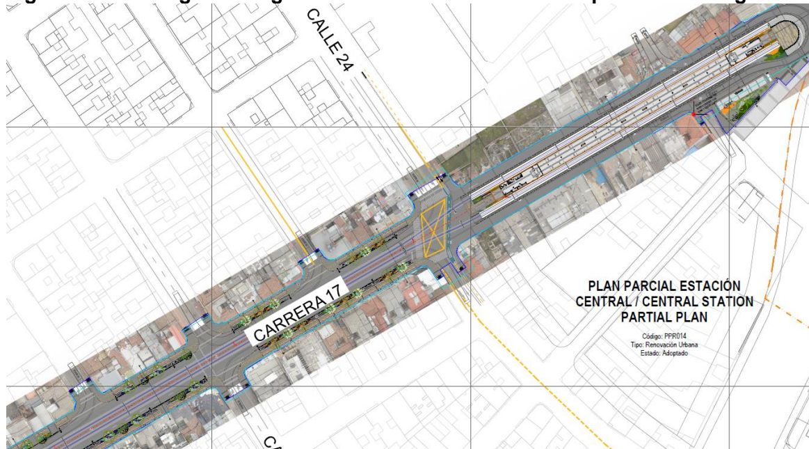
Figura 6-24. Configuración geométrica Carrera 17 x Calle 24 por trazado Regiotram
