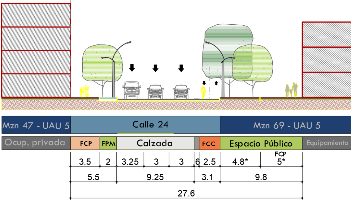
Figura 6-33. Sección transversal Calle 24
