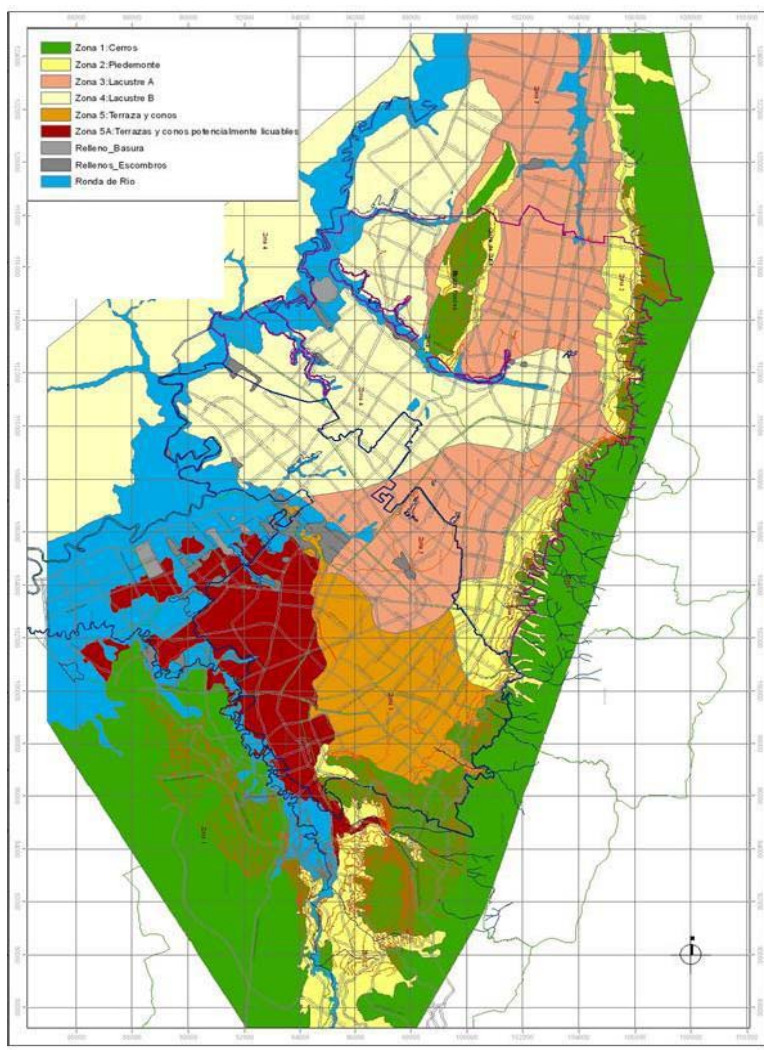
Figura 72. Zonificación Estudio Metro - Microzonificación sísmica de Bogotá
